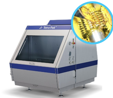
利乐®均质机
